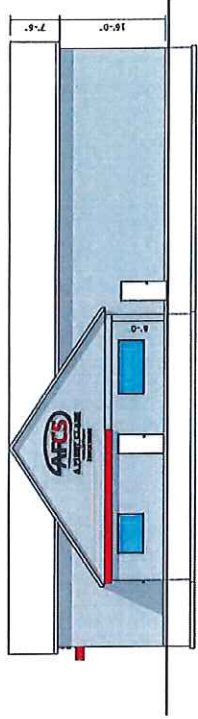
Right Elevation
